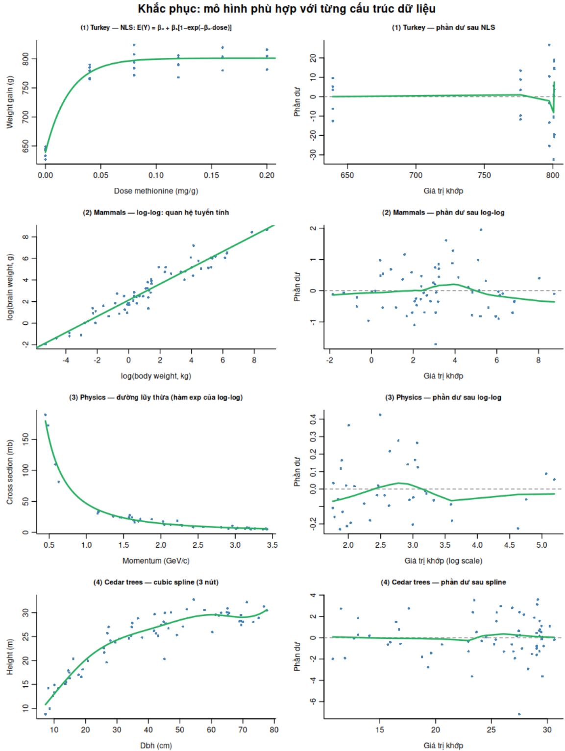
Hình 6: Cùng bốn bộ dữ liệu sau khi áp dụng mô hình phù hợp (xanh lá). (1) Turkey: NLS với dạng bão hòa \beta_0 + \beta_1[1 - e^{-\beta_2 \cdot \text{dose}}] —phần dư trở nên ngẫu nhiên. (2) Mammals: OLS trên thang log-log—quan hệ tuyến tính, phần dư phân tán đều. (3) Physics: khớp lũy thừa qua log-log—phần dư không còn mẫu hình. (4) Cedar trees: cubic spline với 3 nút—đường cong bám sát toàn vùng, phần dư ngẫu nhiên.
